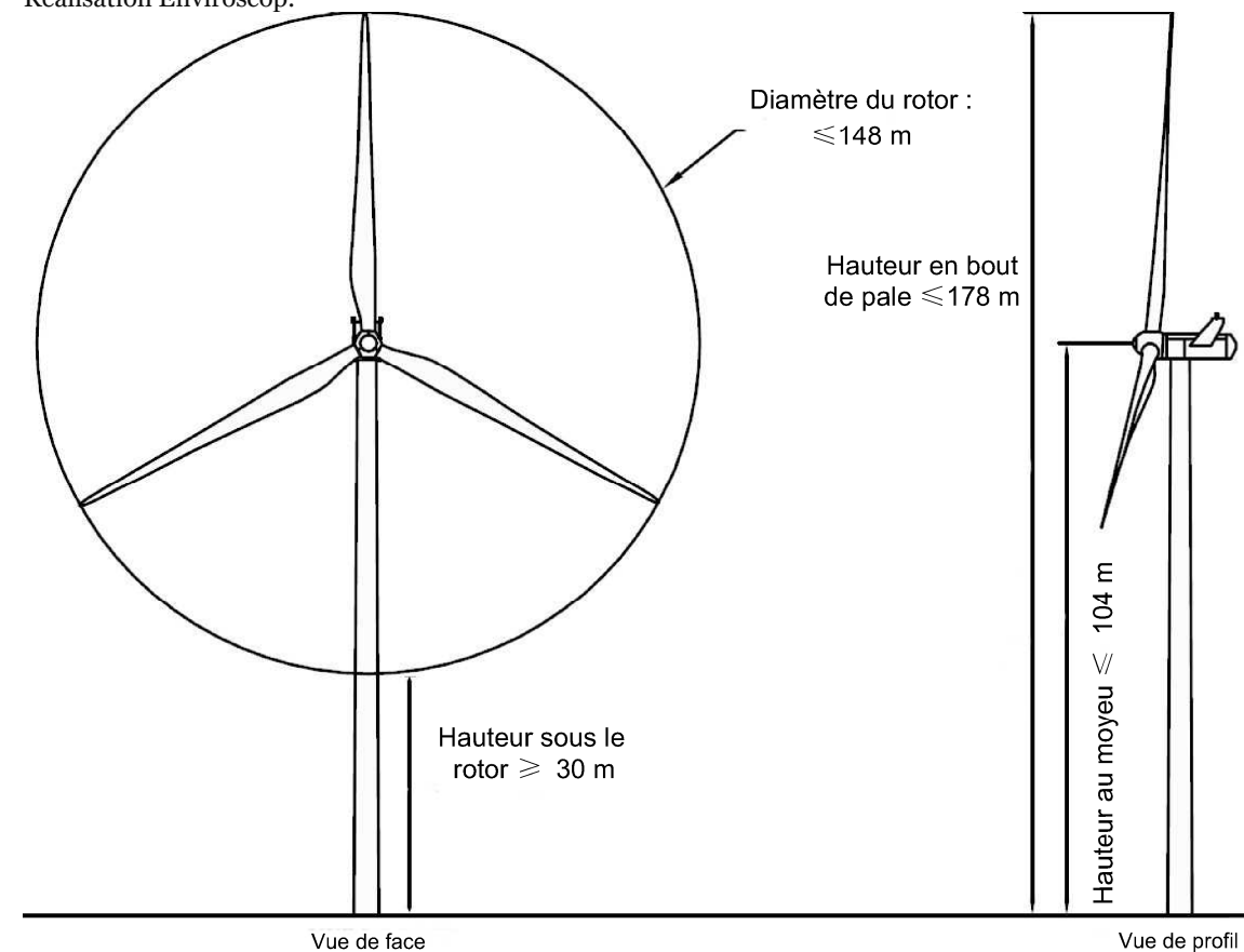
Figure 3 : Vue d'ensemble du gabarit pour l'éolienne E2
