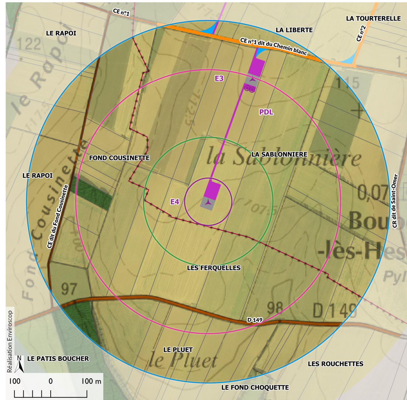
Carte 15 : Synthèse des risques de l'éolienne E4
