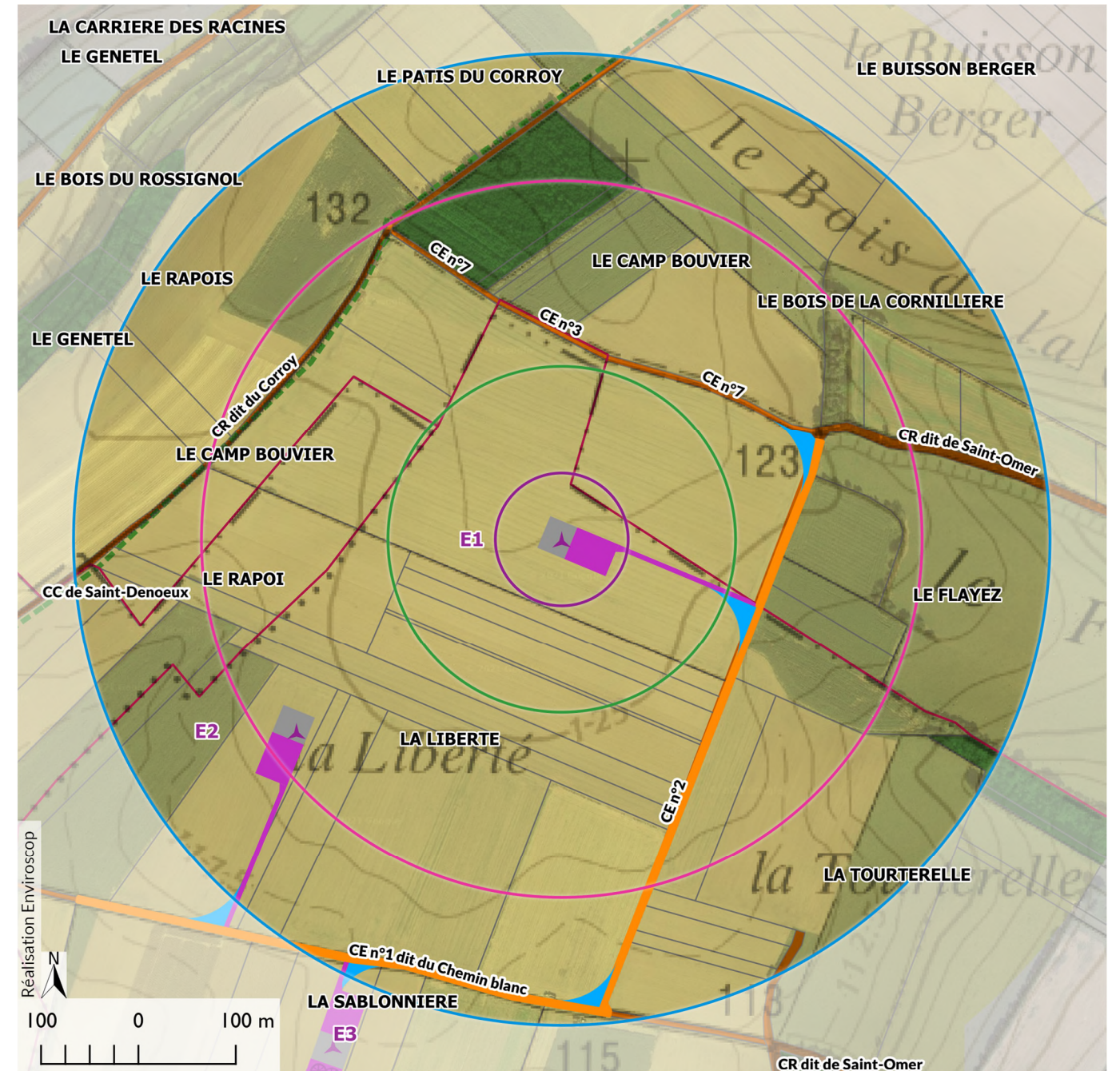
Carte 12 : Synthèse des risques de l'éolienne E1
