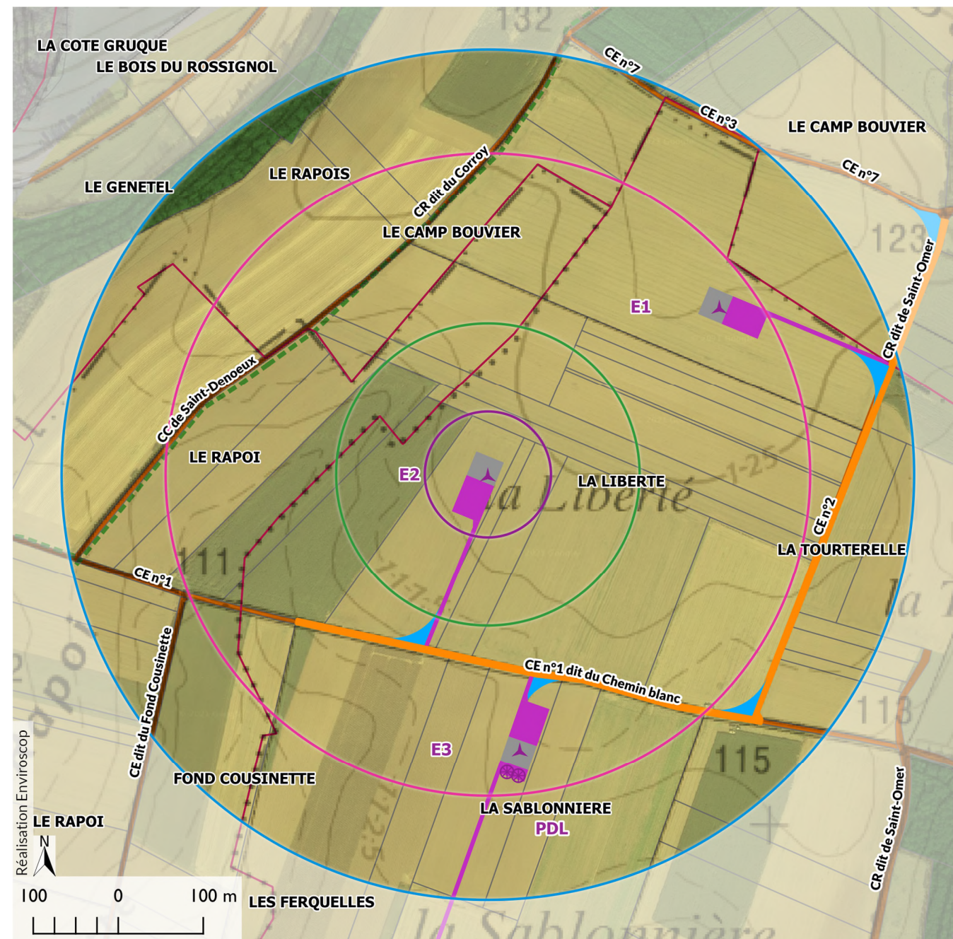
Carte 13 : Synthèse des risques de l'éolienne E2
