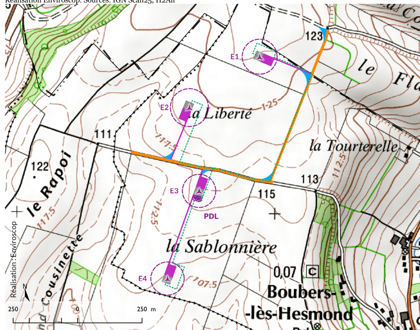
Carte 11 : Plan simplifié du parc éolien des Magnolias
