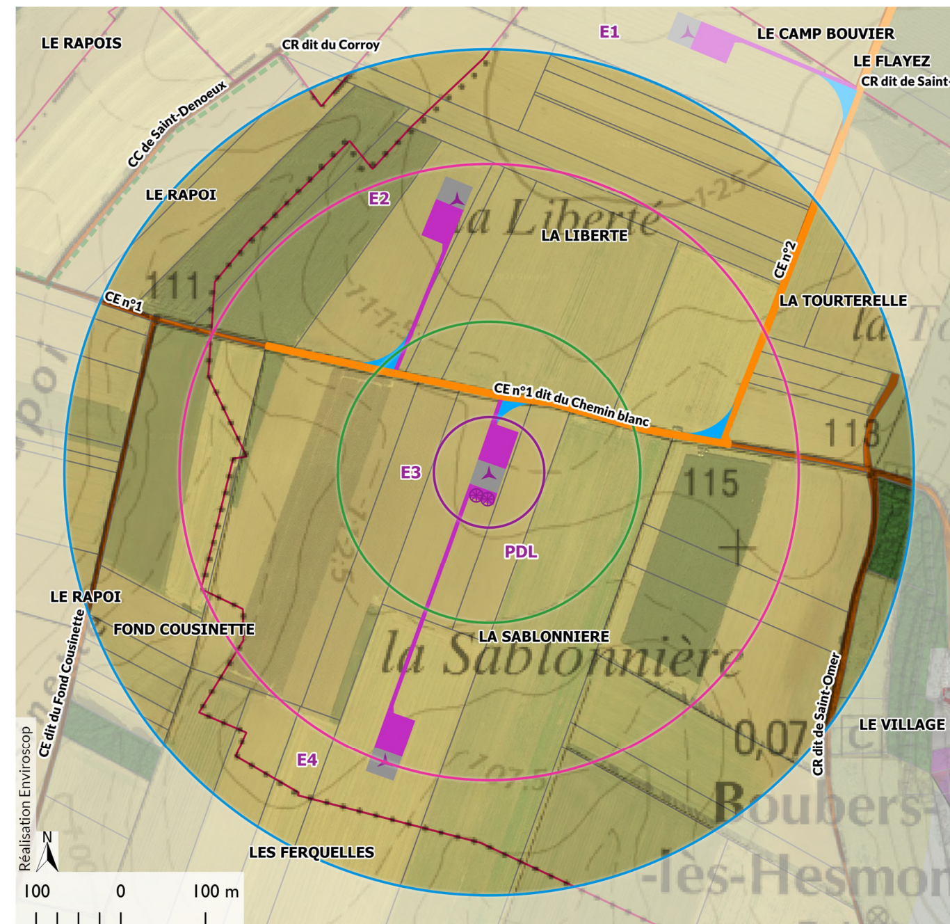
Carte 14 : Synthèse des risques de l'éolienne E3
