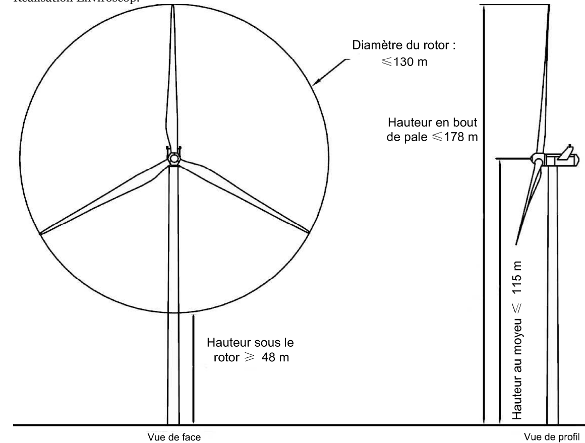
Figure 4 : Vue d'ensemble du gabarit pour les éoliennes E3 et E4
