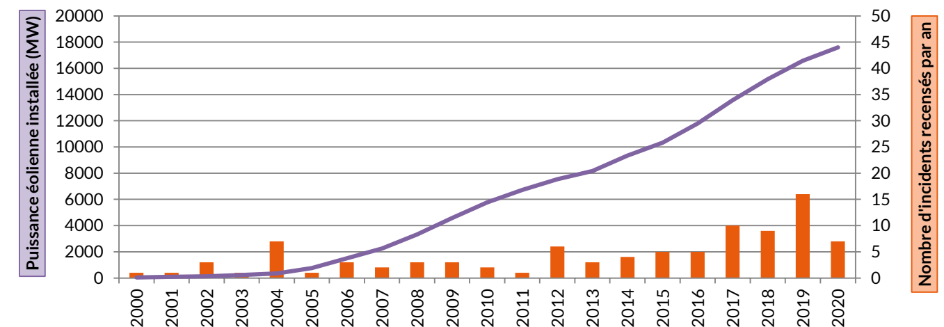
Evolution du nombre d'incidents annuels en France et puissance éolienne cumulée raccordée
