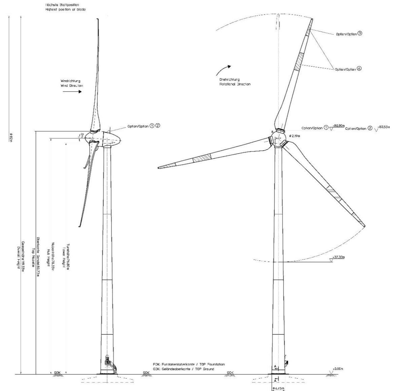
Figure 8 : Vue générale de la E82-78,33 m (source : ENERCON, 2015)
